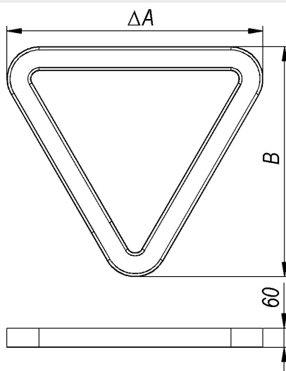
Габаритні розміри.
